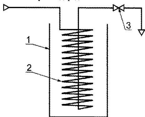
1 — сосуд для охлаждающей смеси; 2 — змеевик; 3 — игольчатый вентиль
