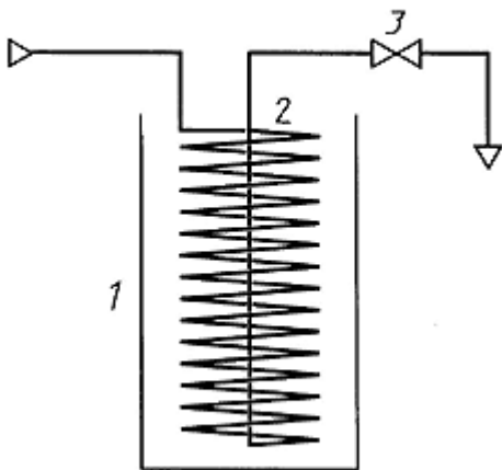
1 — сосуд для охлаждающей смеси; 2 — змеевик; 3 — игольчатый вентиль
